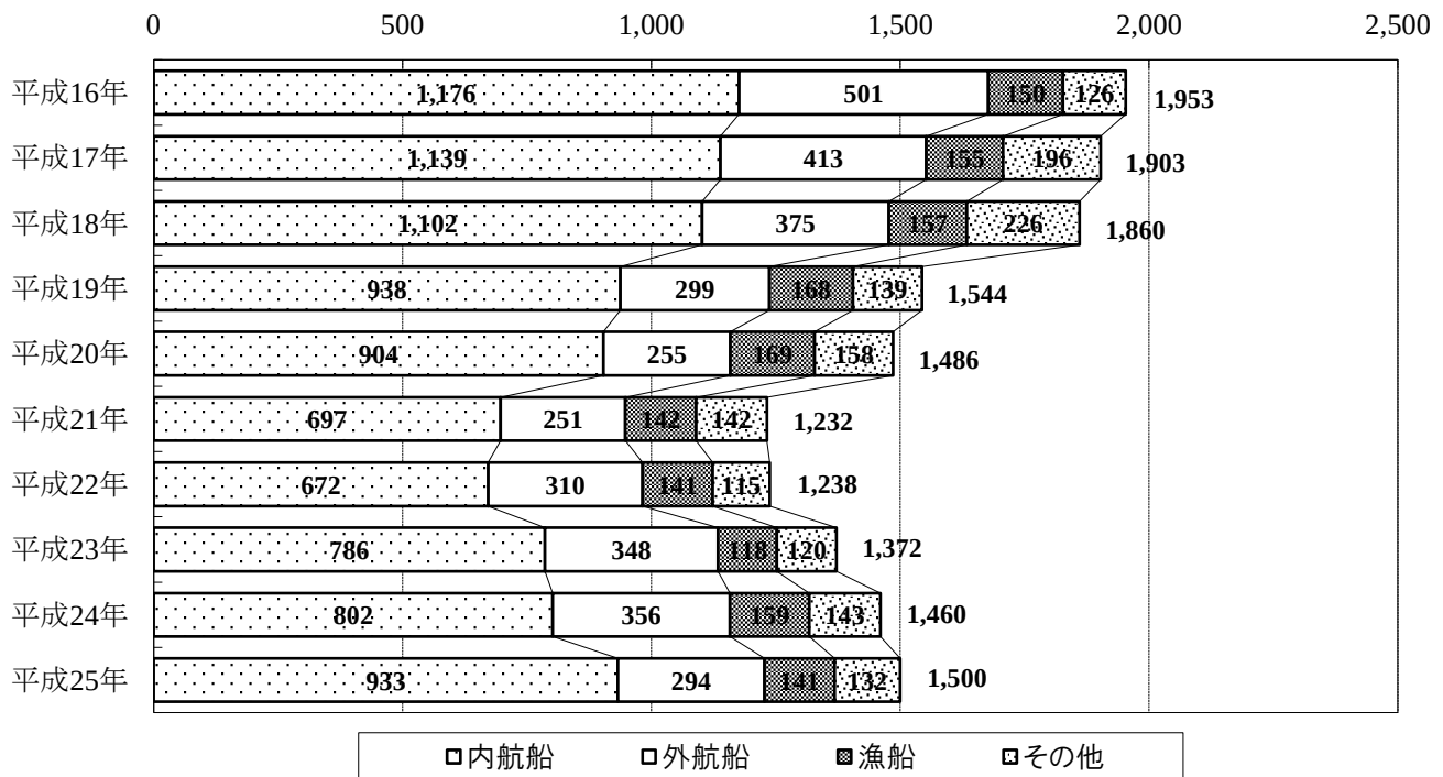
■入港船舶隻数の推移(過去10年間) (単位:隻)
