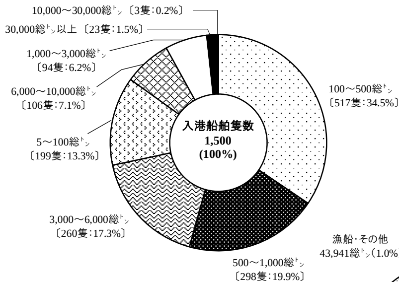
■トン数階級別隻数
